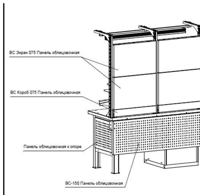
ВС Короб панель облицовочная 075/100 400 руб./ 500 руб.
