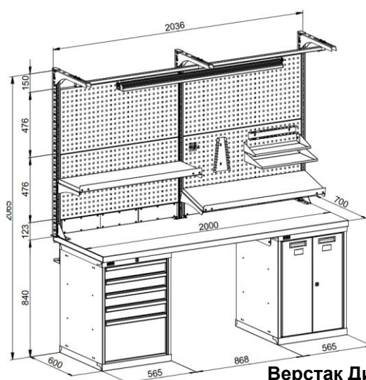
Верстак ДиКом ВС-150
