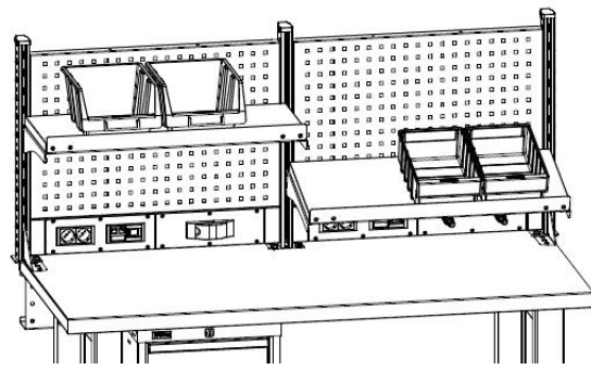
ВС Полки на экран можно установить прямо или под наклоном 15°
