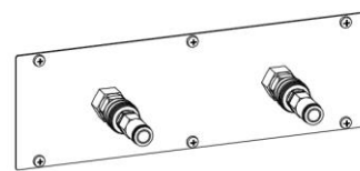
Вставка с 2 пневматическими БРС и цанговыми фитингами (шланг 10) 5 950 руб.
